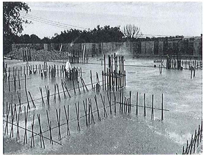
一樓地坪養護
