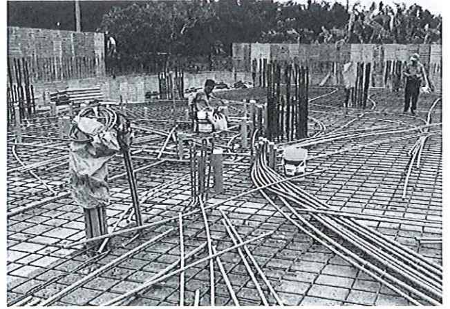
消防及水電管線預埋
